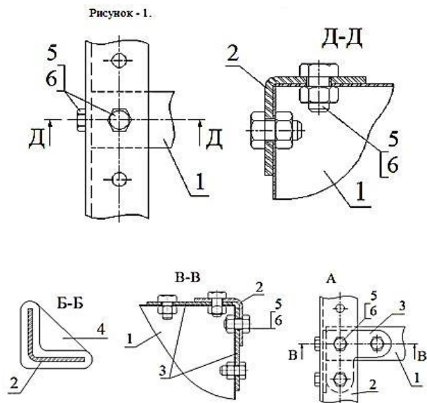
Крепление дополнительной полки без усиливающих уголков
