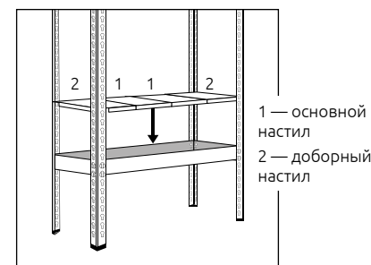
Рис. 5а. Укладка металлического настила
